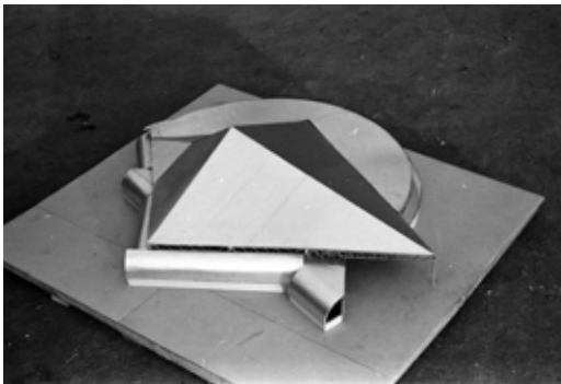
FIG. 2.25 Model of the San José de Arauco Parish. 1962. Source: Archivo Histórico José Vial Armstrong e[ad] PUCV.
